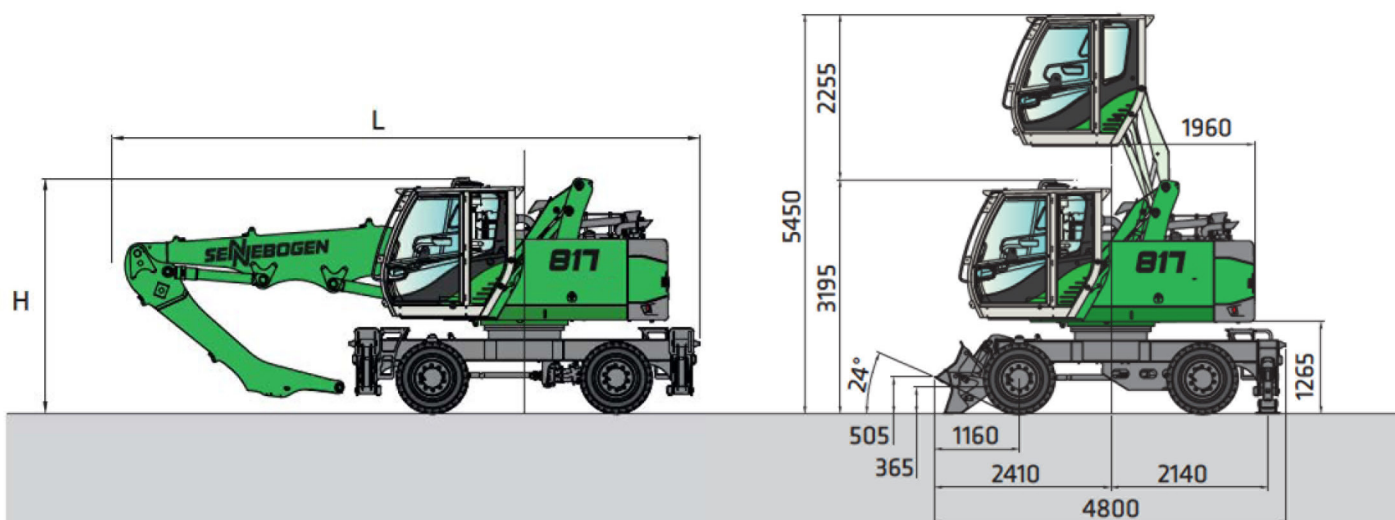
817M с ходовой частью типа MP17
