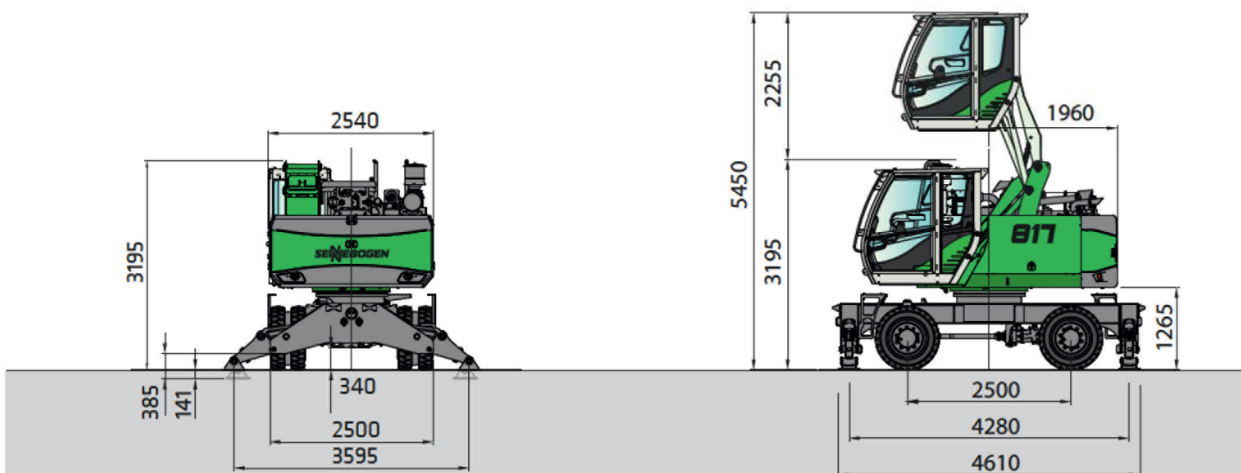
817M с ходовой частью MP17 и кабиной типа E240 с гидравлическим подъемником
